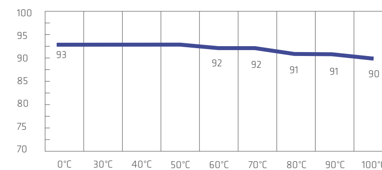
硬度与温度的关系表 ( Shore A)
